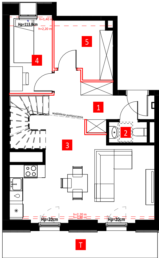
PIĘTRO +6
